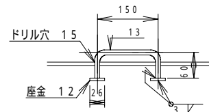
取手詳細図
