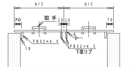
取手詳細図
